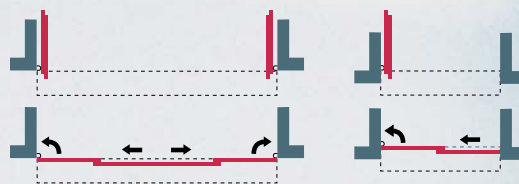
API doble 2 hojas correderas 2 hojas semi-fijas
